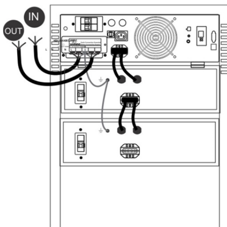
شکل ۱۵- الف: یوپی‌اس SDC6000X-RT PLUS با دو کابینت
