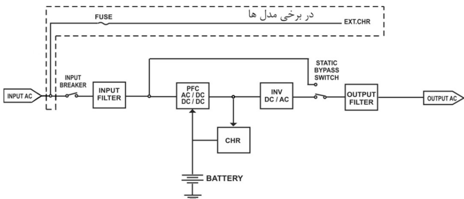
شکل ۳۱: ساختار داخلی یوپی‌اس‌های SDC6000X-RT PLUS
