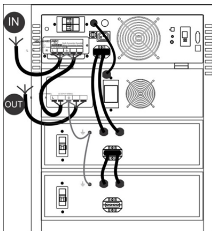
شکل ۱۵- ب: یوپی‌اس SDC6000X-RT PLUS ،
