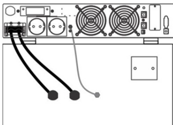
شکل ۹: SDC1000X-RT PLUS و SDC2000X-RT PLUS
