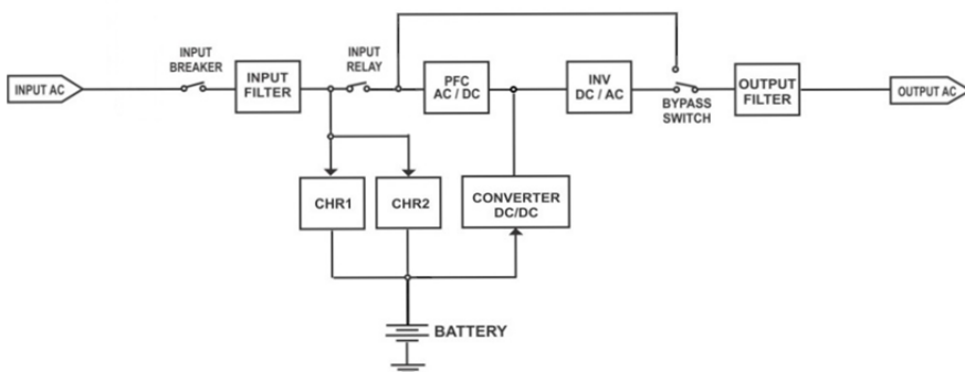
شکل ۲۸: ساختار داخلی یوپی‌اس‌های SDC2000X-RT PLUS
