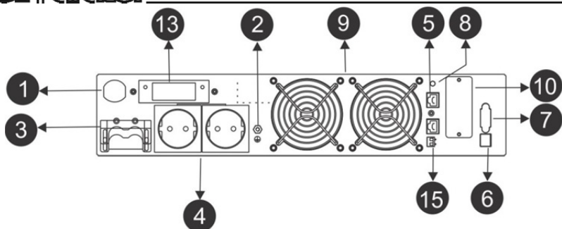
شکل ۳: نمای پنل پشت SDC1000,2000-PLUS
