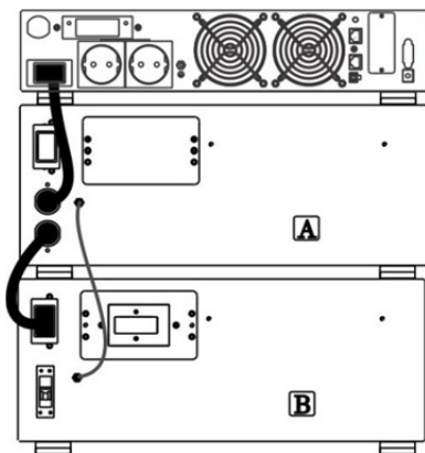
شکل ۸: SDC3000X-RT PLUS
