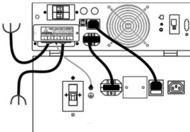
شکل ۱۰: SDC6000X-RT PLUS
