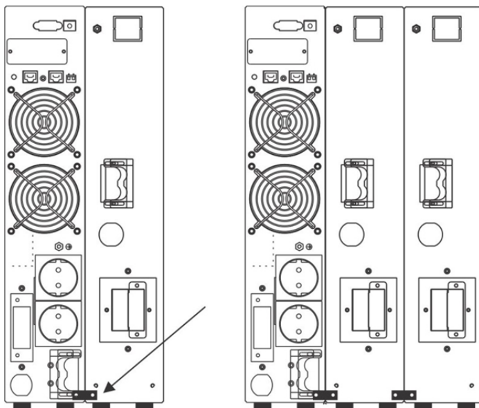
شکل ۱۹: نحوه قرار گرفتن بست‌های نگهدارنده در پشت یوپی‌اس و کابینت باتری
