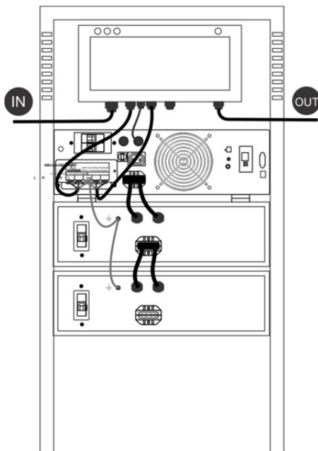
شکل ۱۵- ج: یوپی اس SDC6000X-RT PLUS ، ترانسفورمر
