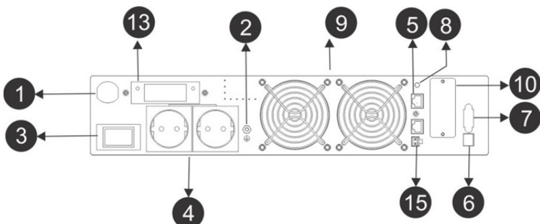
شکل ۴: نمای پنل پشت SDC3000 PLUS
