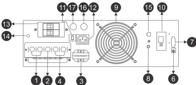
شکل ۵: نمای پنل پشت SDC6000 PLUS
