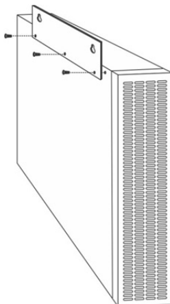
شکل ۲۱: مونتاژ قطعه آویز به SDC2000BW PLUS
