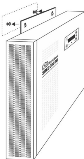
شکل ۲۲: نصب SDC2000BW PLUS بر روی دیوار
