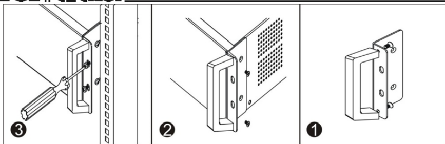
شکل ۱۳: اتصال دستگیره‌های مدل رک
