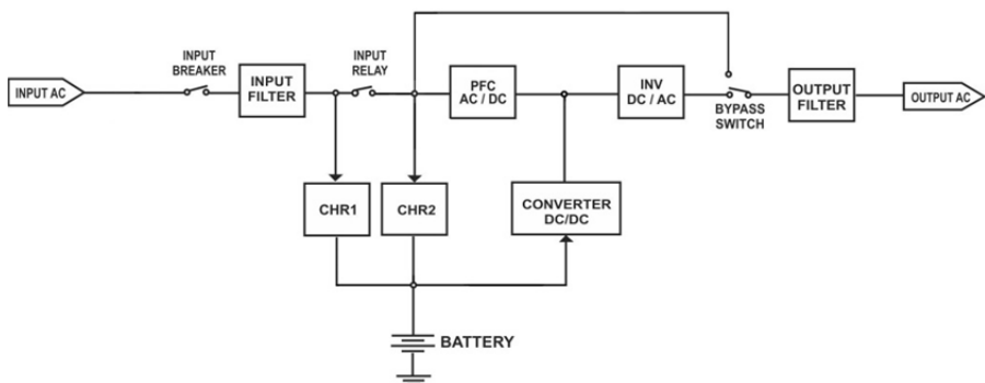
شکل ۳۰: ساختار داخلی یوپی‌اس‌های SDC3000X-RT PLUS
