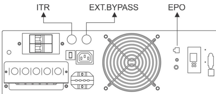
شکل ۲۷: شکل پنل پشت و اتصالات مربوط به ترانسفورمر ایزوله، تابلوی بای پس و EPO
