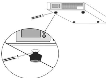
شکل ۱۱: خارج نمودن پایه‌های پلاستیکی
