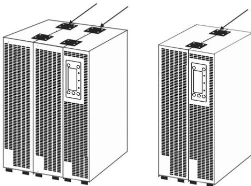
شکل ۱۸: نحوه قرار گرفتن بست‌های نگهدارنده بر روی یوپی‌اس و کابینت باتری
