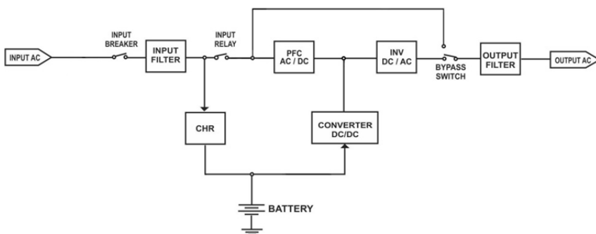
شکل ۲۹: ساختار داخلی یوپی‌اس‌های SDC2000BW PLUS ، SDC1000X-RT PLUS
