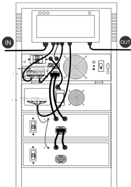
شکل ۱۵- د: یوپی اس SDC6000X-RT PLUS ،
