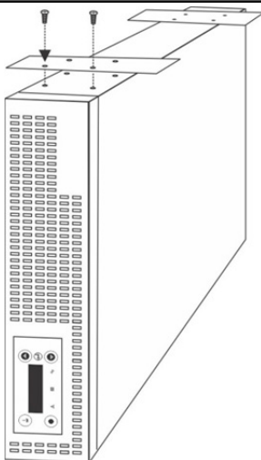
شکل ۲۳: بستن پلتهای فلزی به SDC2000B-RT PLUS
